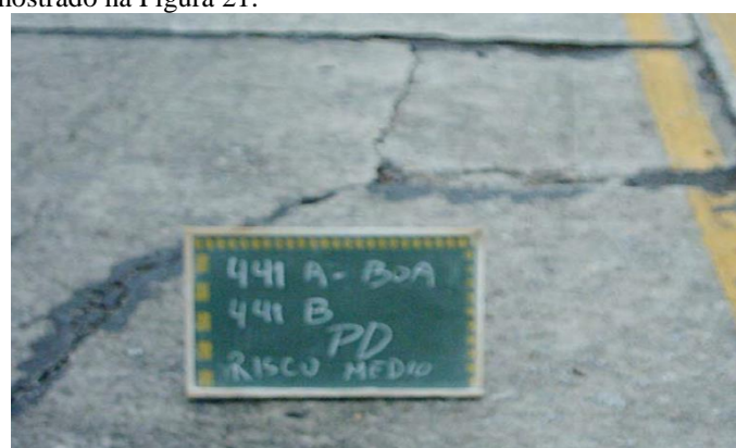
Figura 21: Assentamento. Fonte: DNIT, 061/2004.
