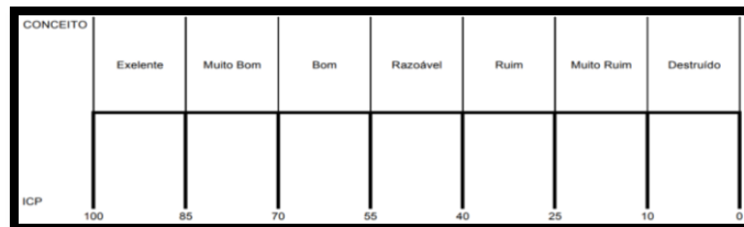
Figura 26: Escala de avaliação do ICP. Fonte: DNIT 062/2004.
