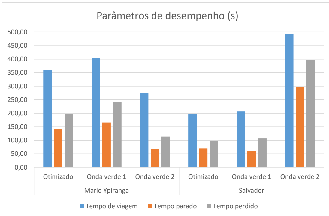
Figura 9: Gráfico com os parâmetros de desempenho. Fonte: Autores, (2017).
